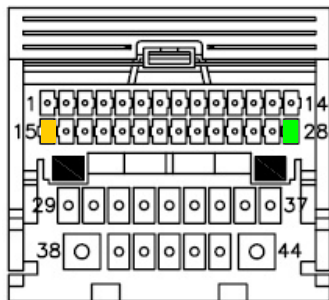
Connettore radio Ingresso cavi Vista posteriore
